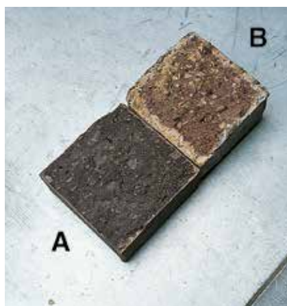
Fot. 1. Próba penetracji jonami chloru (UNI 9944). Próbkę A została zabezpieczona izolacją Mapelastic i nie wykazuje penetracji; próbka B, bez izolacji wykazuje zniszczenia różnej wielkości.
